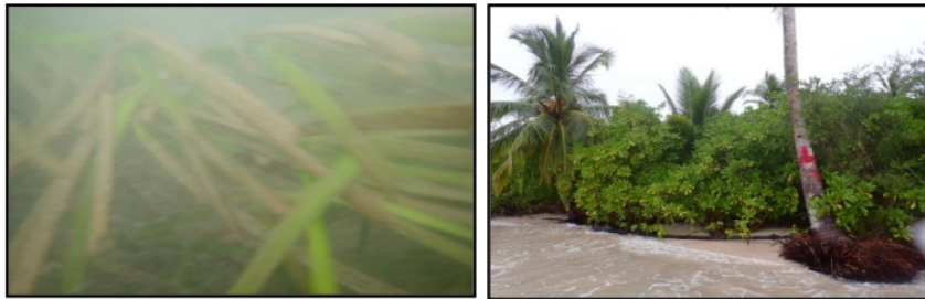
Gambar 3.42. Lokasi MTWL01 dan lamun yang ditemukan didominasi oleh Halodule uninervis .
