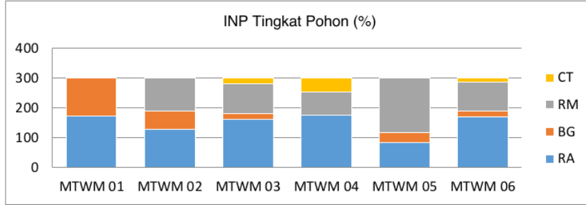
Gambar 3.48. Grafik Nilai INP Tingkat Pohon Setiap Stasiun pengamatan
