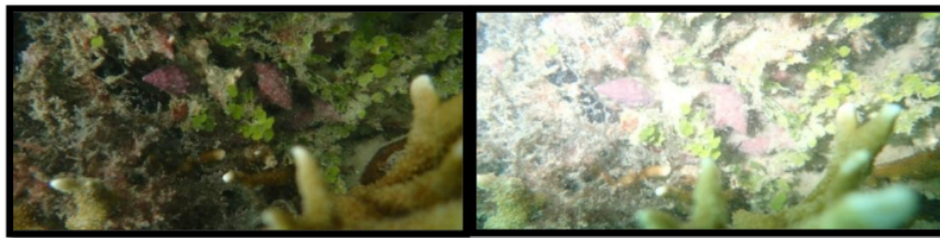
Gambar 3.34 Beberapa Siput Drupella spp. yang ditemukan di TWP Selat Bunga Laut
