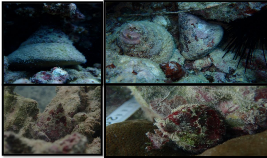
Gambar 3.38. Beberapa keong trokha yang ditemukan di TWP Selat Bunga Laut
