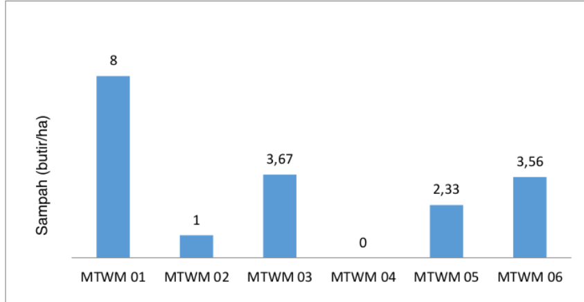
Gambar 3.57. Jumlah Sampah yang Ditemukan pada Setiap Stasiun Pengamatan
