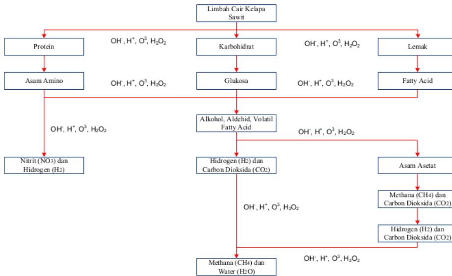
Gambar 5.1 Proses penguraian POME dengan metode
