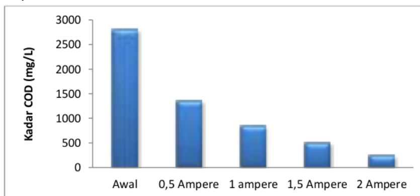
Gambar 4.5 Pengaruh arus terhadap kadar COD
