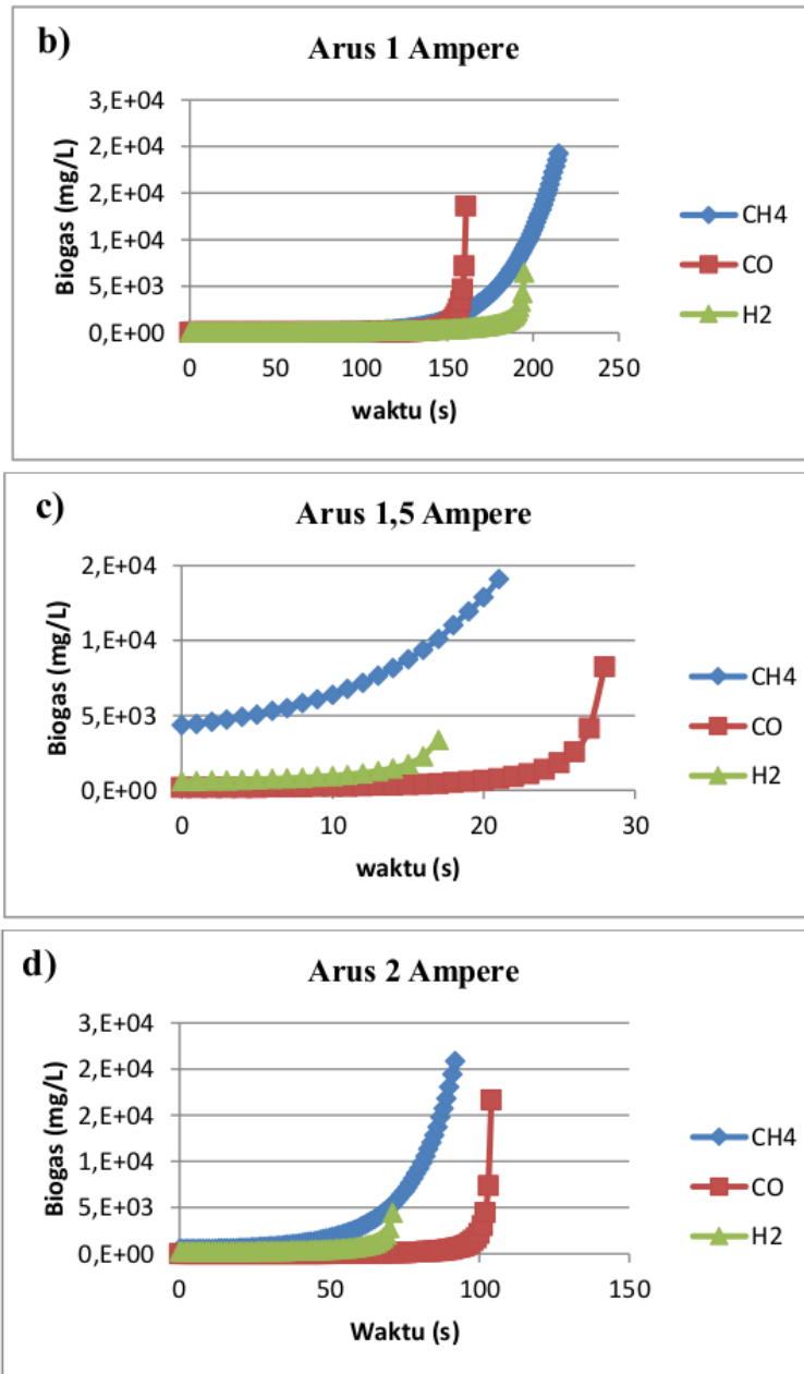
Gambar 4.3 Profil biogas terhadap waktu
