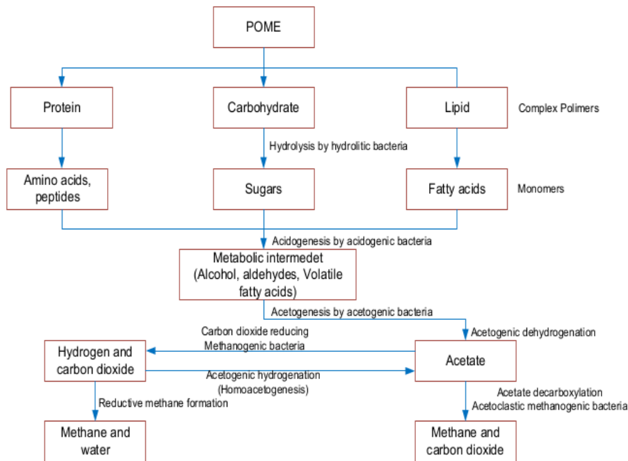
Gambar 2.1 Proses Penguraian POME menjadi biogas secara anaerobik Sumber : (Ohimain & Izah, 2017)
