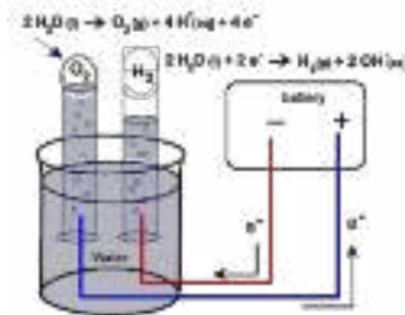
Gambar 4.1 Komponen Sel elektrolisis
