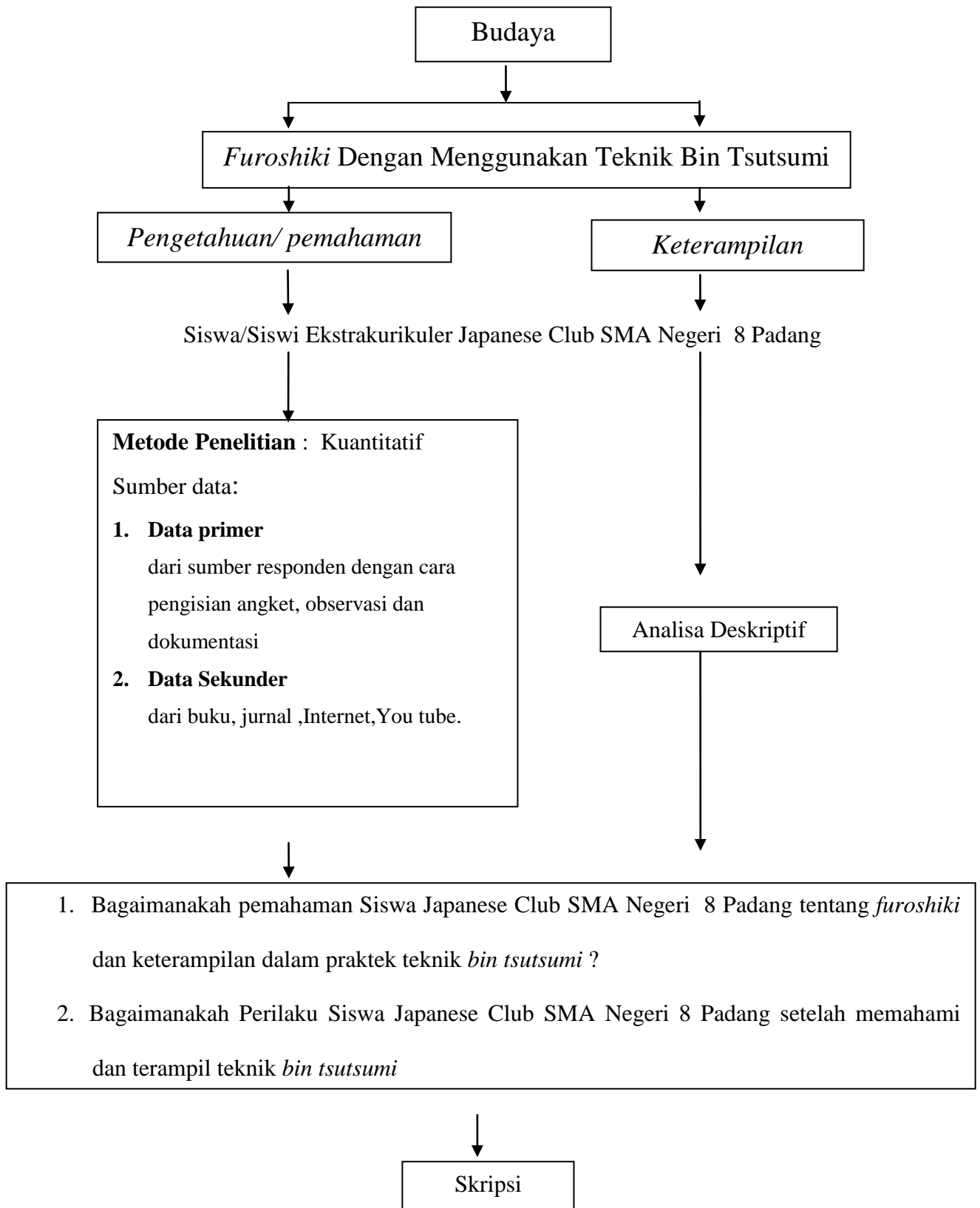
Gambar 1 Kerangka Konseptual
