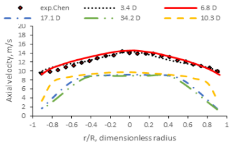
a). Axial velocity profile.
