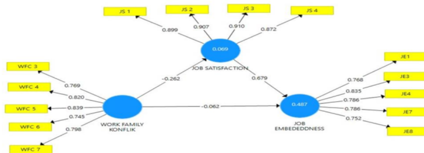
Gambar 1 Pengaruh X dan Y Melalui Terhadap M (Sumber: Data primer SEM-PLS).
