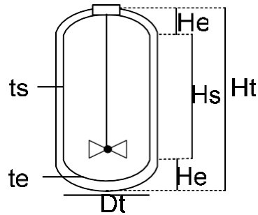
Gambar L-C.7 Tangki Pelarutan Kaporit
