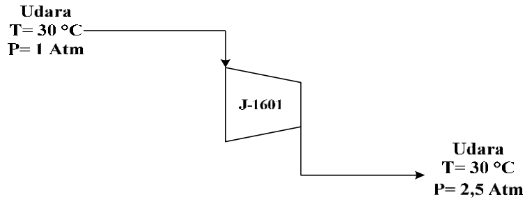
Gambar L-C.1 Kompresor (J-1601)
