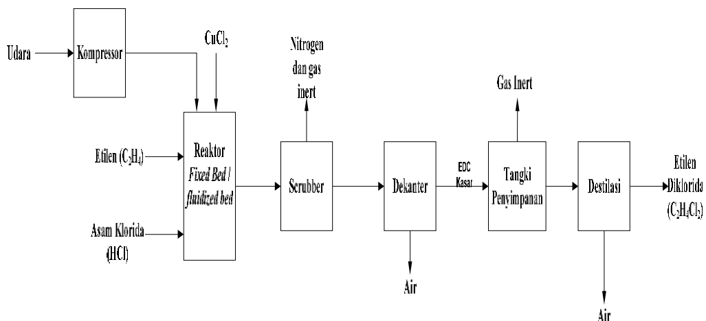
Gambar 2.4. Blok Diagram Proses Oksiklorinasi
