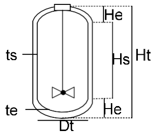
Gambar L-C.6 Tangki Pelarutan Alum
