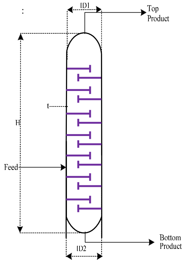
Gambar L-C.7 Kolom Destilasi
