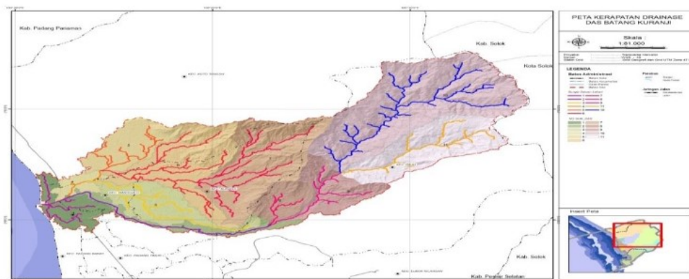
Gambar 3. Kerapatan Drainase
