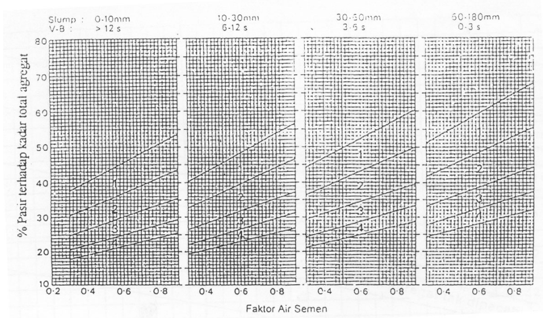
Grafik 14 Persen pasir perhadap kadar total agregat yang dianjurkan untuk ukuran butir maksimum 20 mm
