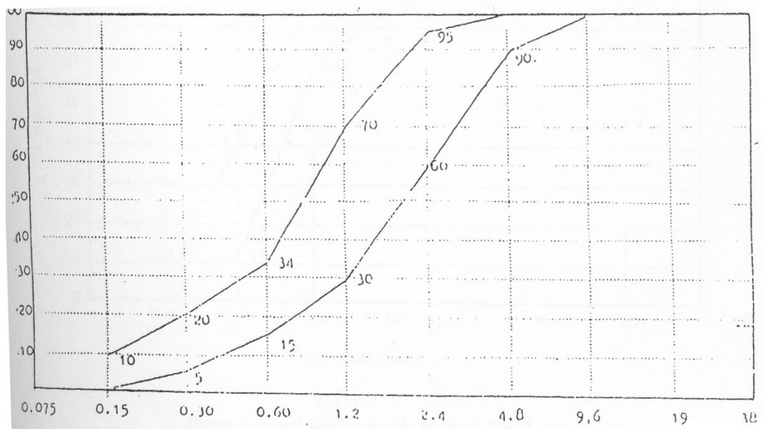
Grafik 3 Batas gradasi pasir (Kasar) No. 1
