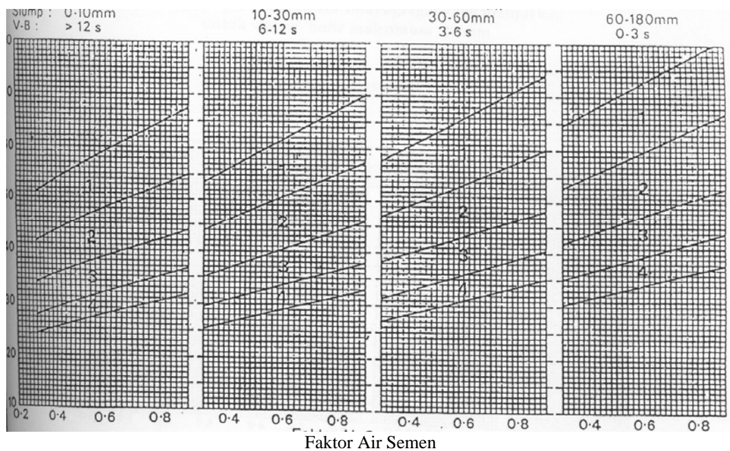
Grafik 13 Persen pasir terhadap kadar tola agregat yang dianjurkan Untuk ukuran butir maksimum 10 mm
