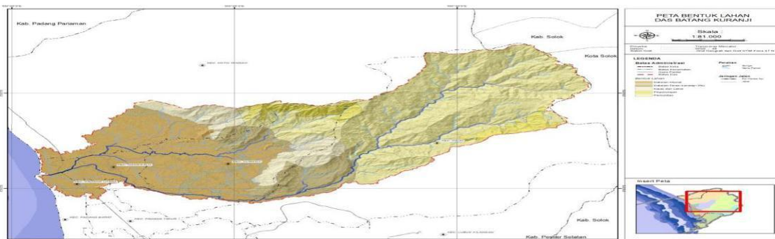
Gambar 9. Bentuk Lahan
