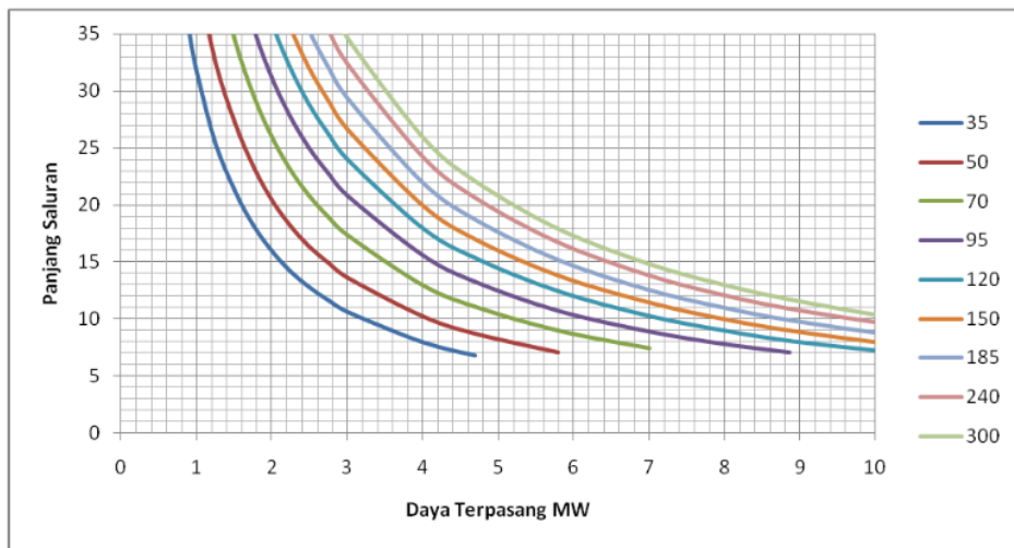
Gambar 4.3 Pemilihan Ukuran Kawat Penghantar SUTM 20 kV dengan drop Tegangan 10%
