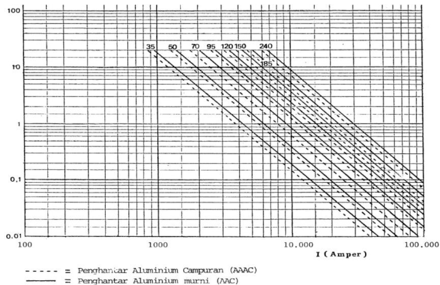
Gambar 3.1 Kurva Kelelahan konduktor A3C dan A2C
