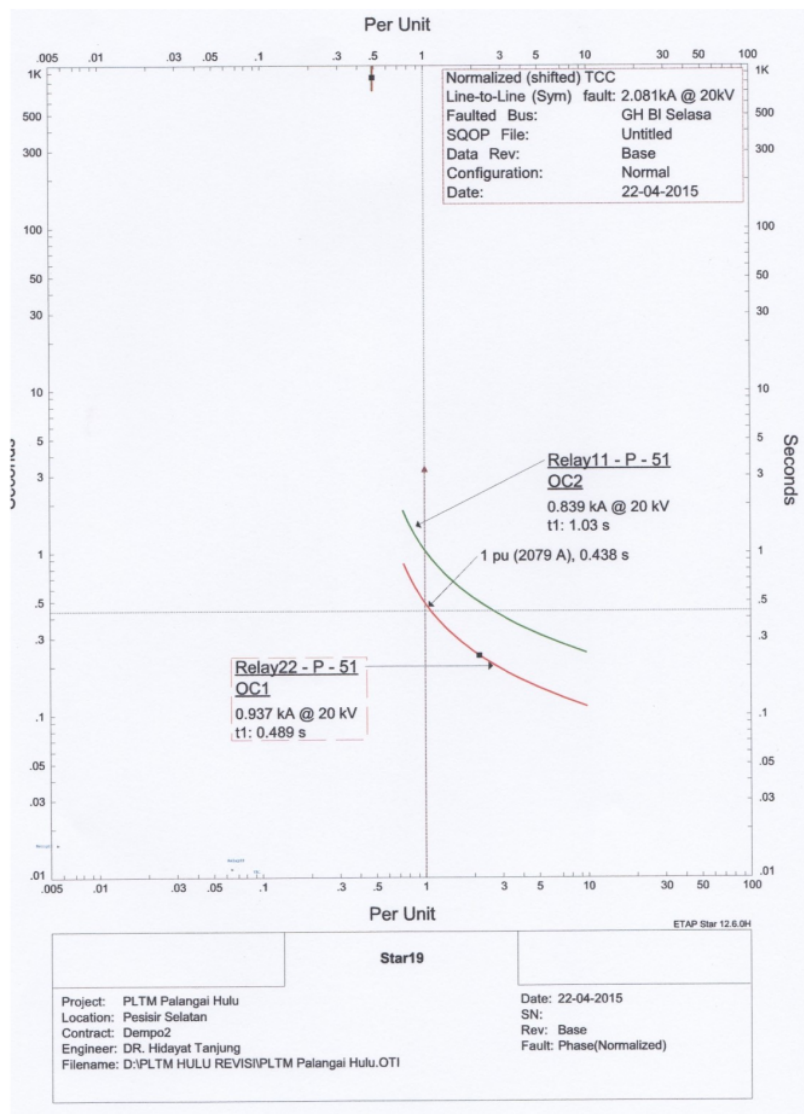
Gambar 3.2 Kurva TOC Relay 11, Relay 22 Saat Gangguan Fasa ke Fasa pada Busbar 20 kV GH Balai Selasa
