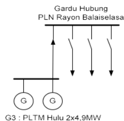
Gambar 4.1 Diagram Segaris PLTM Palangai Hulu
