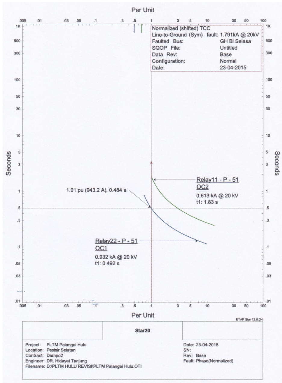
Gambar 3.3 Kurva TOC Relay 11 dan Relay 22 Saat Gangguan Fasa ke Tanah di Bus GH Balai Selasa
