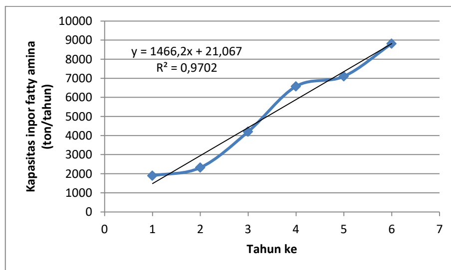
Gambar 1.1 Kurva Kapasitas Impor Fatty amine
